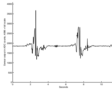
(f) Gyro 3
