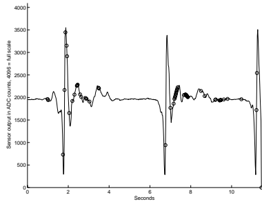
(d) Gyro 1
