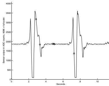
(d) Gyro 1
