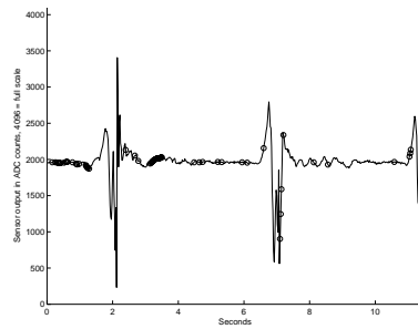
(f) Gyro 3
